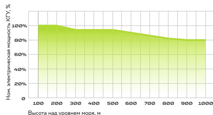
График снижения номинальной мощности КГУ
